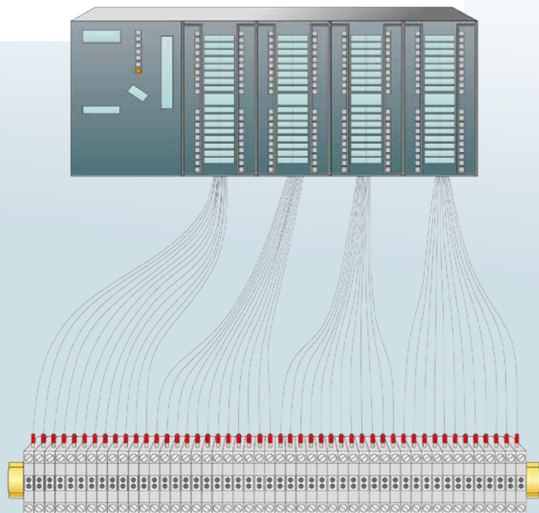
传统布线方式
